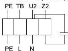
Схема электрических соединений CFk MAX, CFs (1~230 В)
