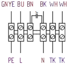
Схема №1 230В, 1ф, 50Гц
