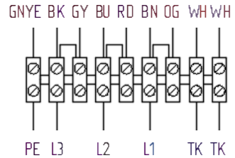
Схема №5 400В, 3ф, 50Г
