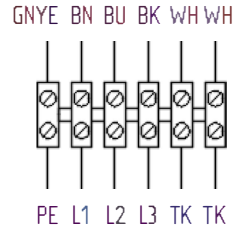
Схема №3 400В, 3ф, 50Г
