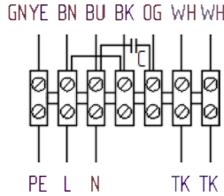
Схема №2 230В, 1ф, 50Гц
