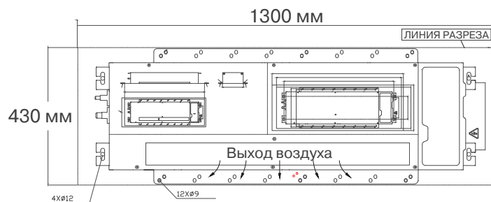
Монтажный шаблон
