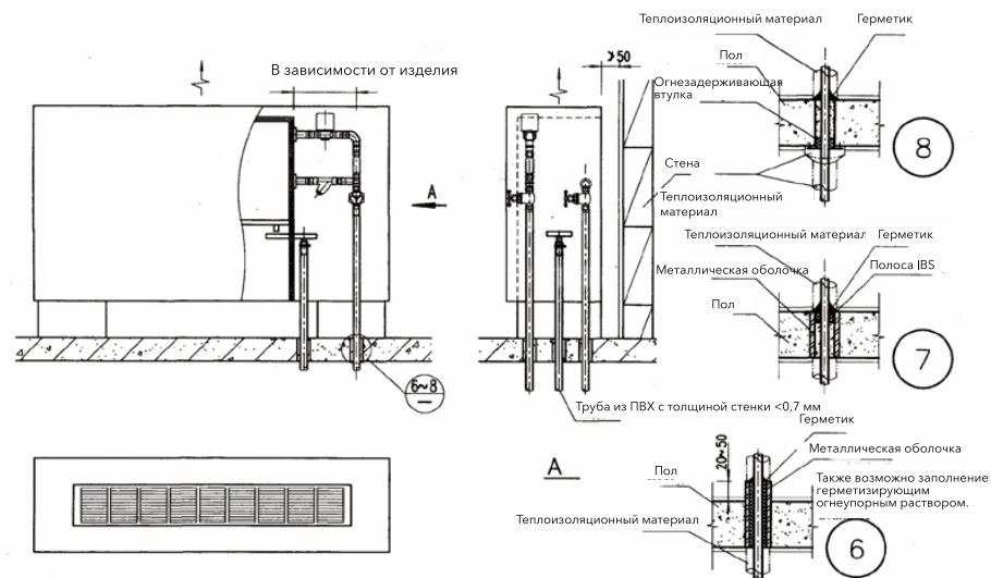
Схема установки вертикального фанкойла
