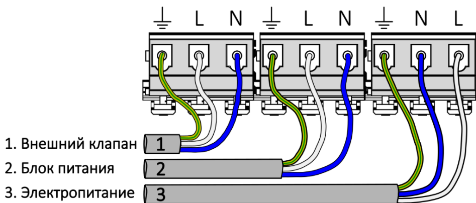
Рис. 4 Клеммная колодка
