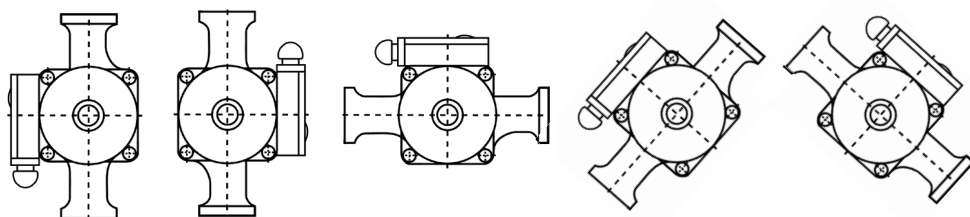
Рис. 8. Возможные варианты монтажа насоса
