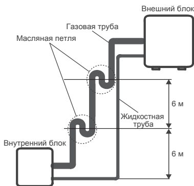
2. Внешний блок установлен выше внутреннего блока
