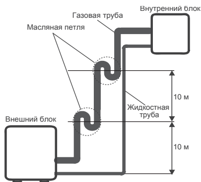
1. Внутренний блок установлен выше наружного блока
