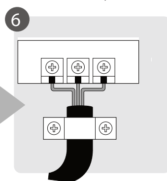
6 Подключите электропроводку
