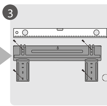
3 Закрепите монтажную пластину
