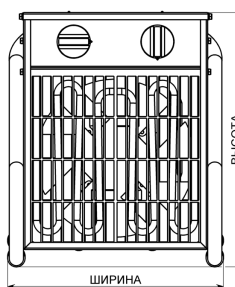
Модели ТПЦ-2, ТПЦ-3, ТПЦ-5, ТПЦ-9, ТПЦ-15, ТПЦ-23, ТПЦ-30
