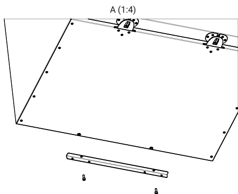
Крепление монтажной планки для установок VRE
