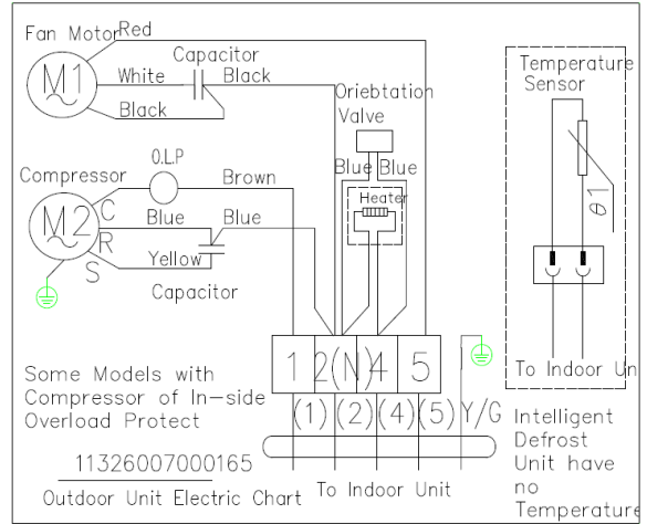
Наружный блок моделей RAS/RAC-07AX,09AX,12AX,18AX
