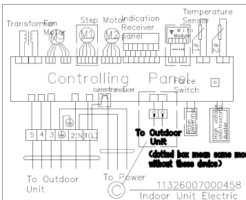
Внутренний блок моделей RAS/RAC-24AX, 30AX, 36AX
