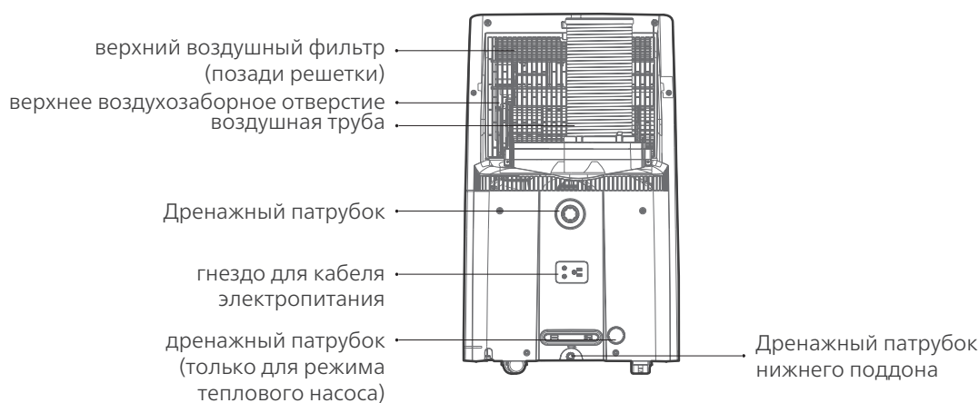
Вид сзади
