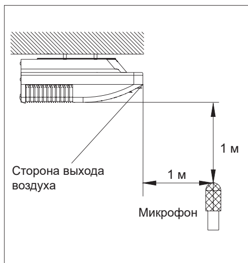
Установка на потолке
