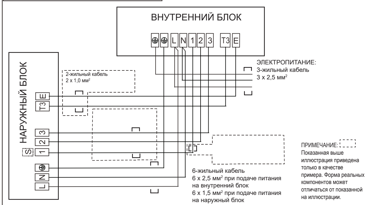
Схема соединений кондиционера
