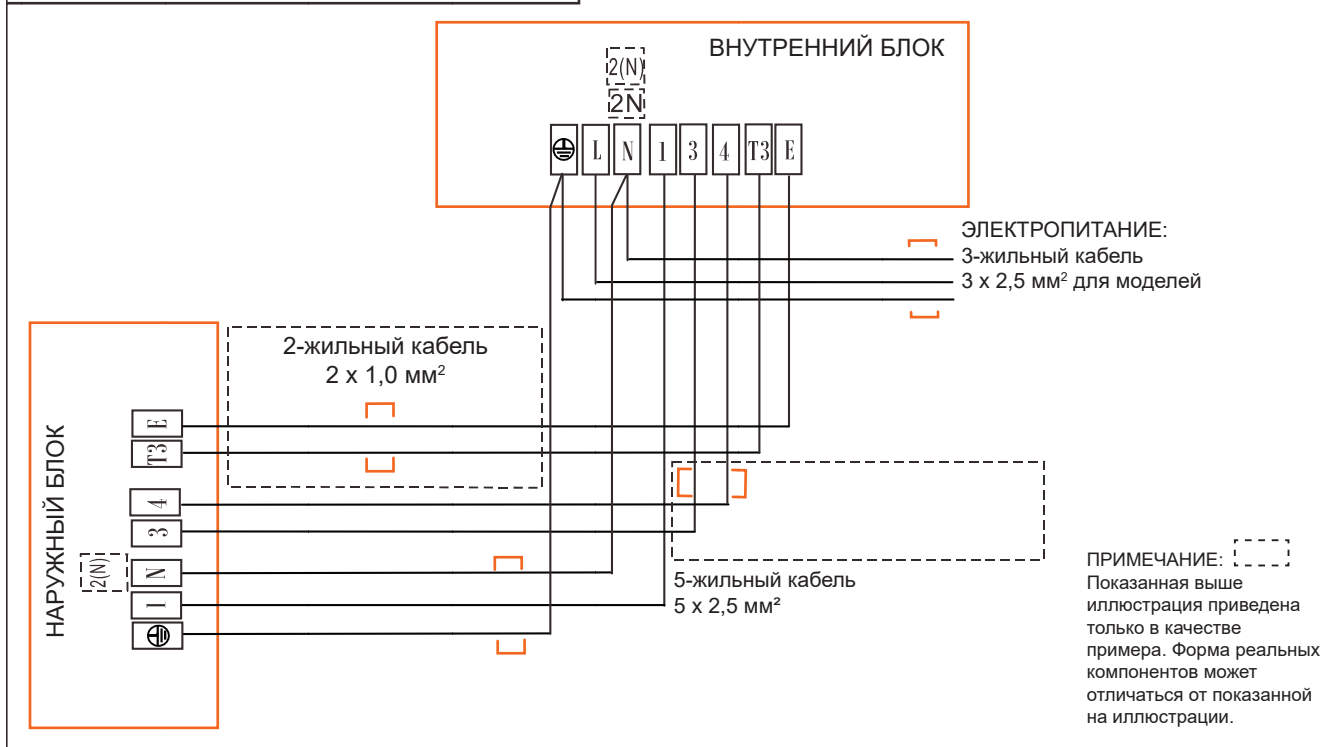
Схема соединений кондиционера
