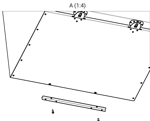
Крепление монтажной планки для установок VRW
