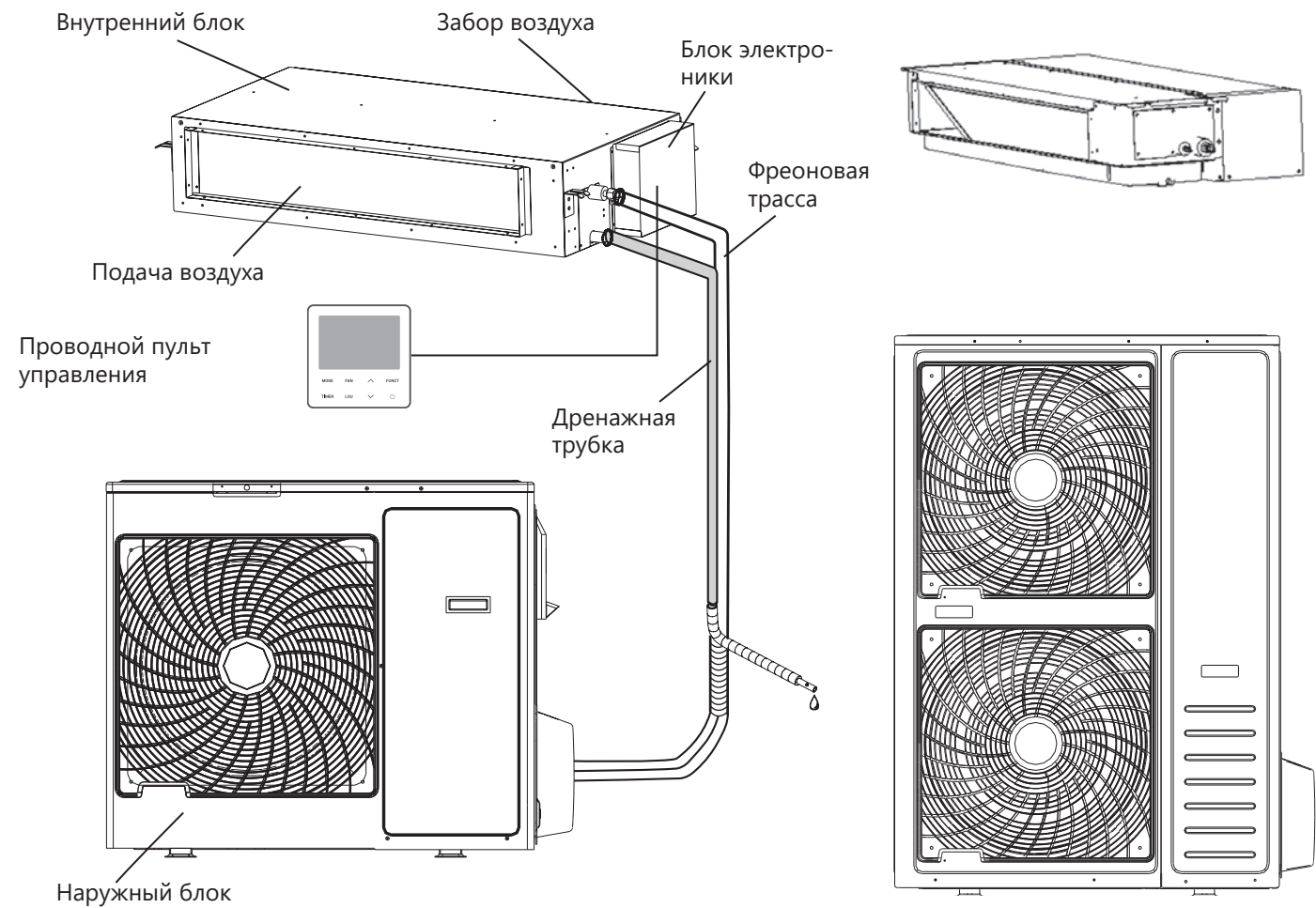
Наружный блок (типоразмер 12/18/24/36)
