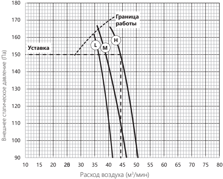
AUD-48HX4REM2/AUD-60HX4REM2(установка 150 Па)
