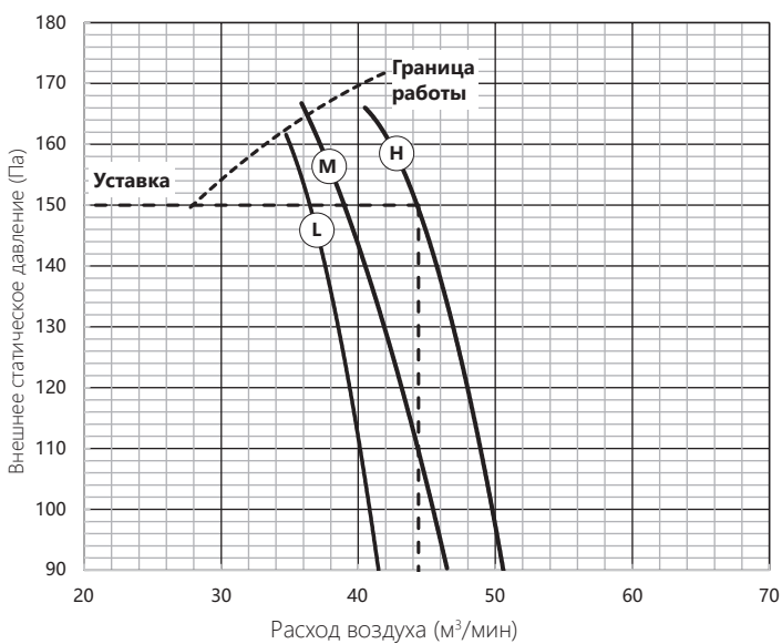
AUD-48HX4REM2/AUD-60HX4REM2(установка 150 Па)
