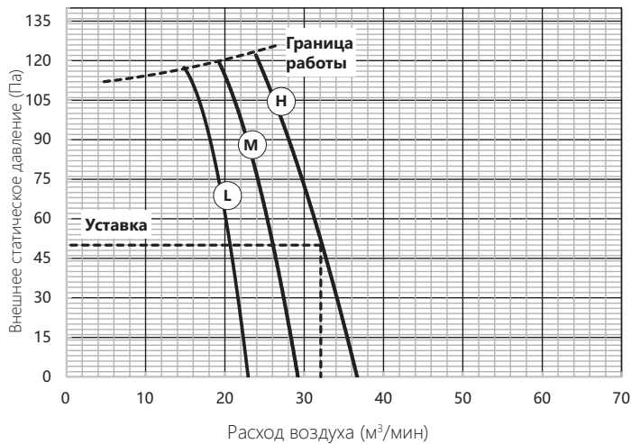
AUD-36HX4RFM2(установка 60 Па)
