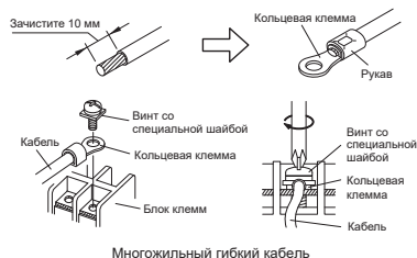
Многожильный гибкий кабель
