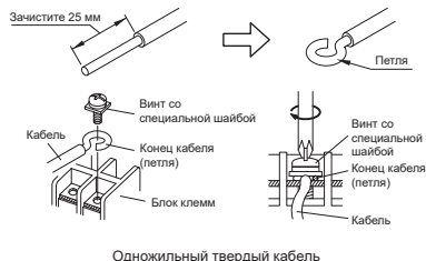
Одножильный твердый кабель
