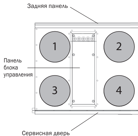
Вид сверху. Установка правого исполнения (по умолчанию)
